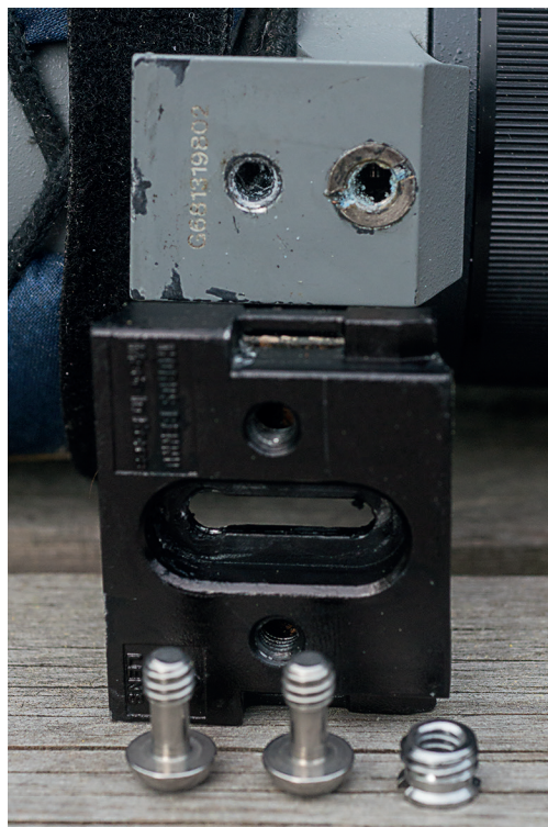
En äldre Swarovskitub med två skruvhål. Ett 1/4" och ett 3/8". Det behövs en övergång från 3/8 till 1/4 för att använda båda skruvhålen. Dessa övergångar säljs i butiker som säljer kameror.
